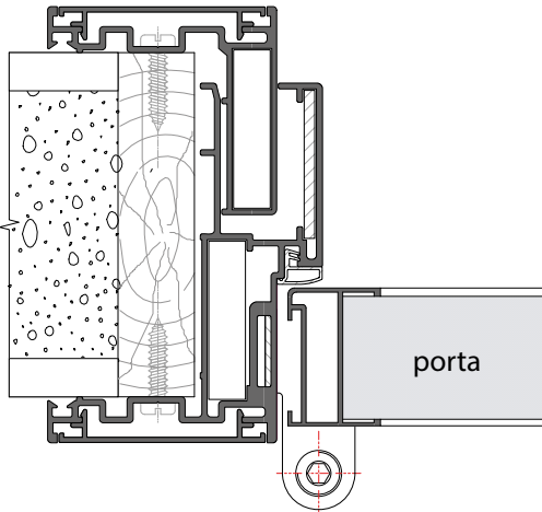
Telaio porta battente profilo linear
