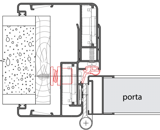
Telaio porta battente profilo standard
